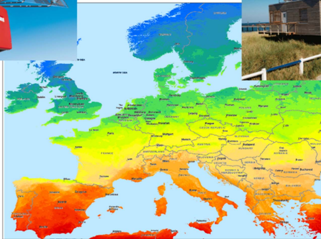
Sonneneinstrahlung 2007 kWh/m 2
